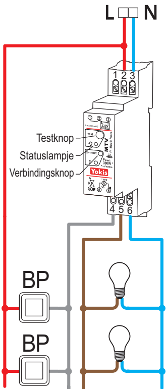
Standaard verbindingsschema
